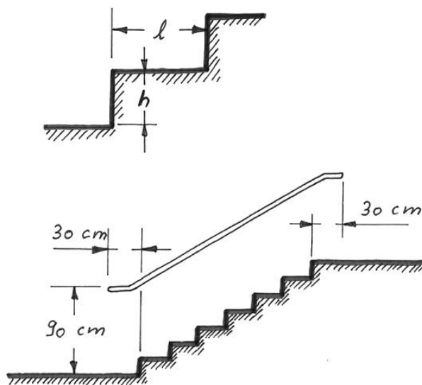
Figure 20 : escalier et mains courantes
