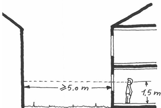
Figure 8 : vues directes et horizontales depuis les pièces destinées au séjour prolongé de personnes vers l'extérieur
