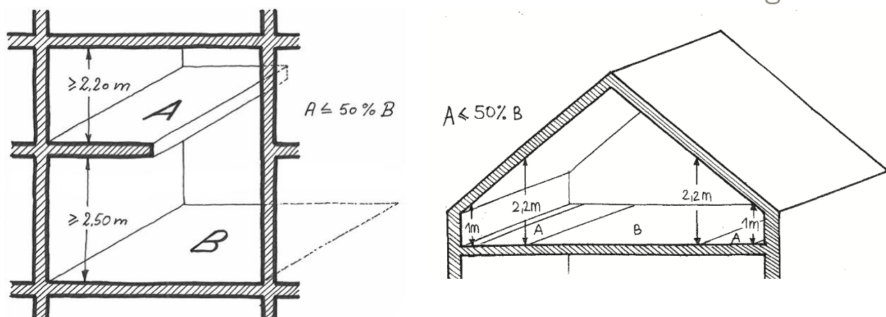
Figure 9 : hauteur libre sous plafond en cas d'une mezzanine ou de combles
