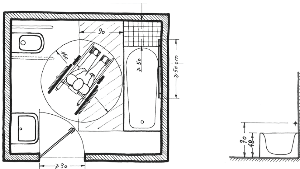
Figure 22 : aménagement d'une salle de bains
