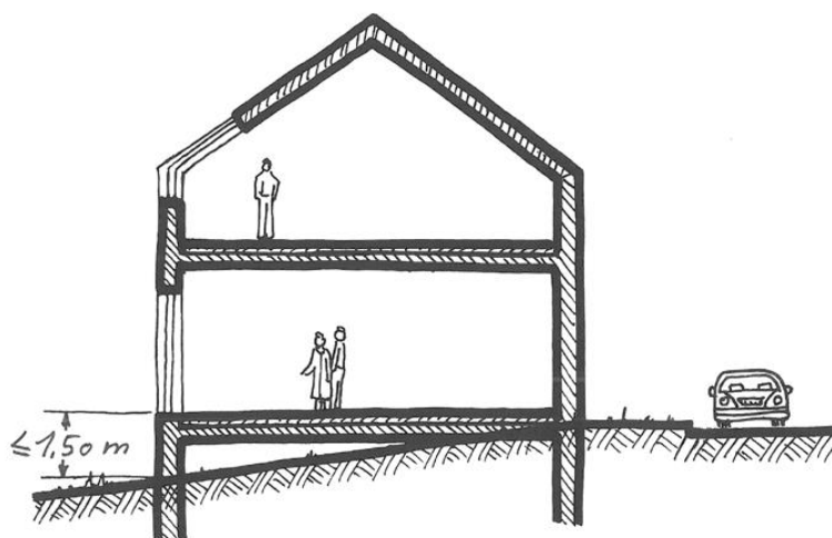
Figure 17 : différence de hauteur entre le terrain naturel et le rez-de-chaussée ou le rez-de-jardin
