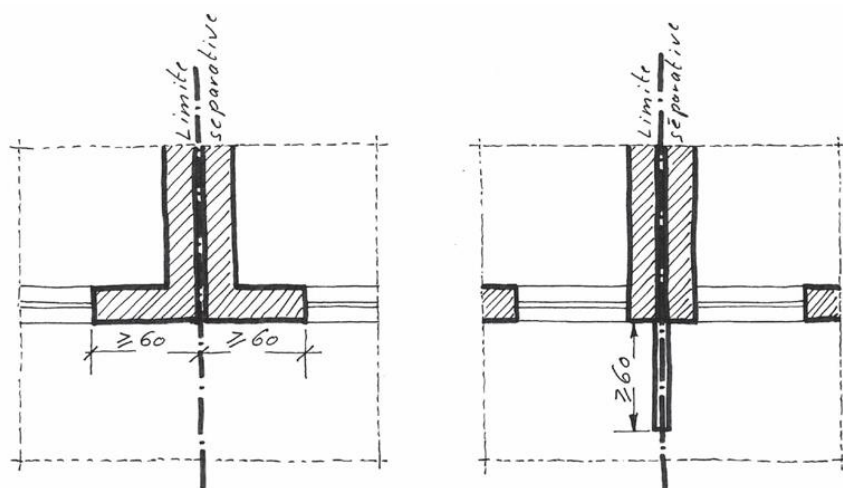
Figure 10 : distance entre ouvertures
