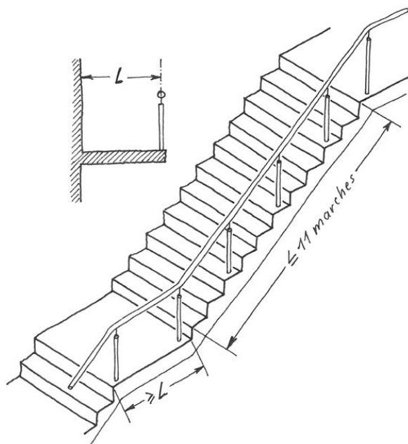
Figure 12 : géométrie d'un escalier
