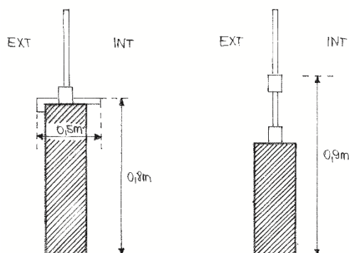
Figure 17 : hauteurs allèges
