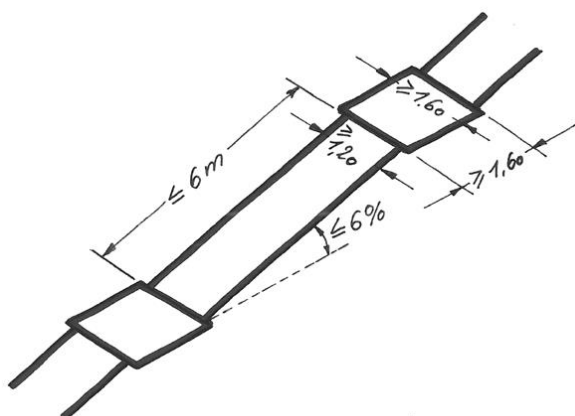
Figure 18 : plan incliné
