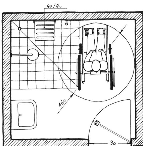
Figure 23 : aménagement d'une cabine de douche
